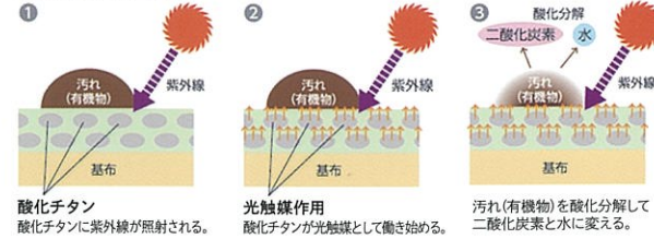
光触媒防汚メカニズム
